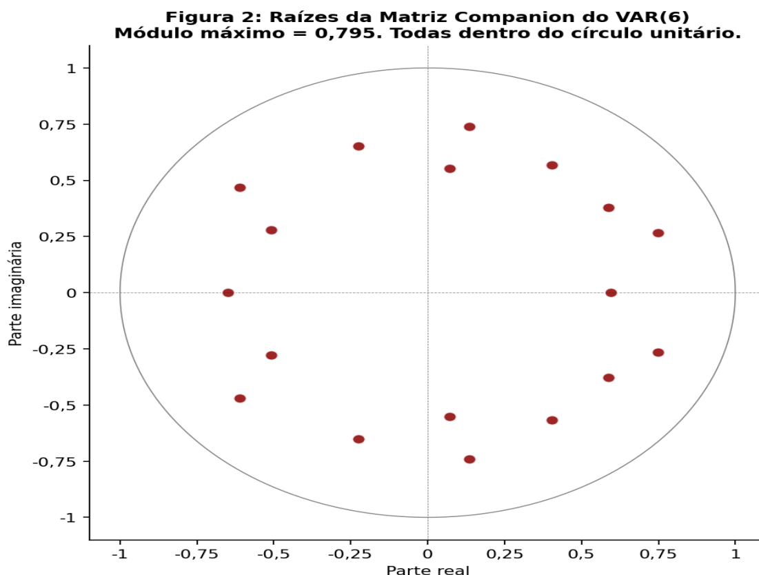
Figura 2: Raízes da Matriz Companion do VAR(6).
