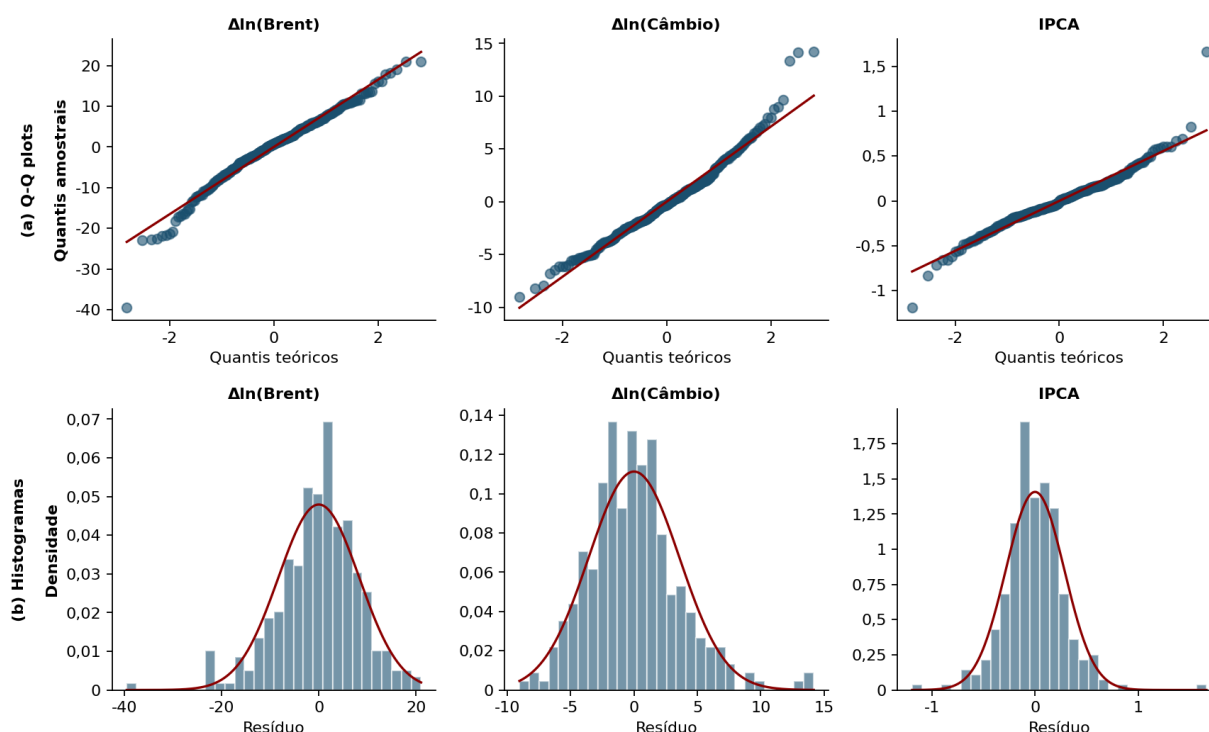
Figura 3: Diagnóstico dos Resíduos do VAR(6) – Q-Q plots e histogramas.
