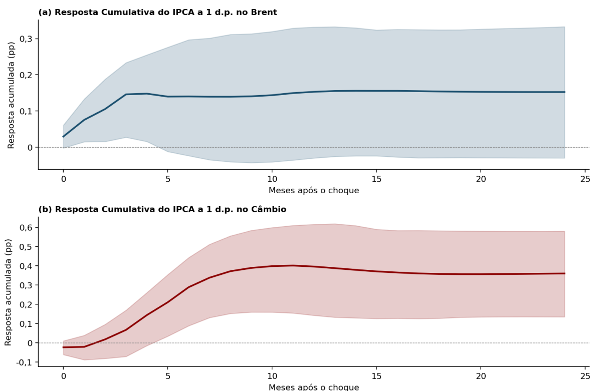
Figura 5: IRFs Cumulativas do IPCA. Bandas de 95% por bootstrap (500 replicações).
