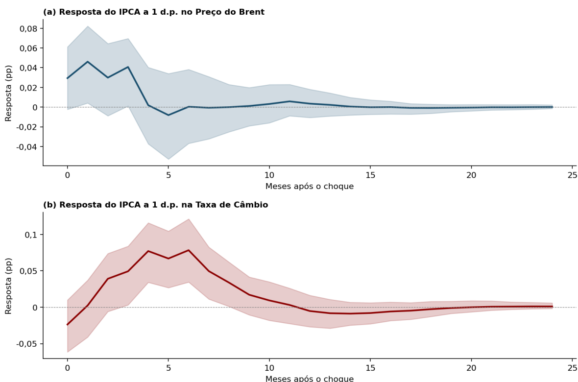
Figura 4: Funções de Impulso-Resposta do IPCA. Bandas de 95% por bootstrap (500 replicações).
